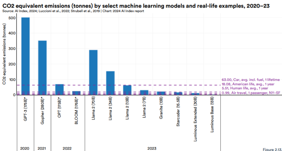
Fig. 2.17. Émissions en tonnes équivalentes CO2 des LLM, extrait de 2024 AI index Report de Stanford [59].
